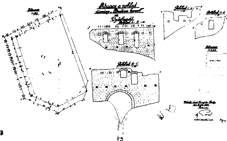
Obr. 2. Praha 2, Vyšehrad. Libušína lázeň — zaměření objektu z roku 1924.
