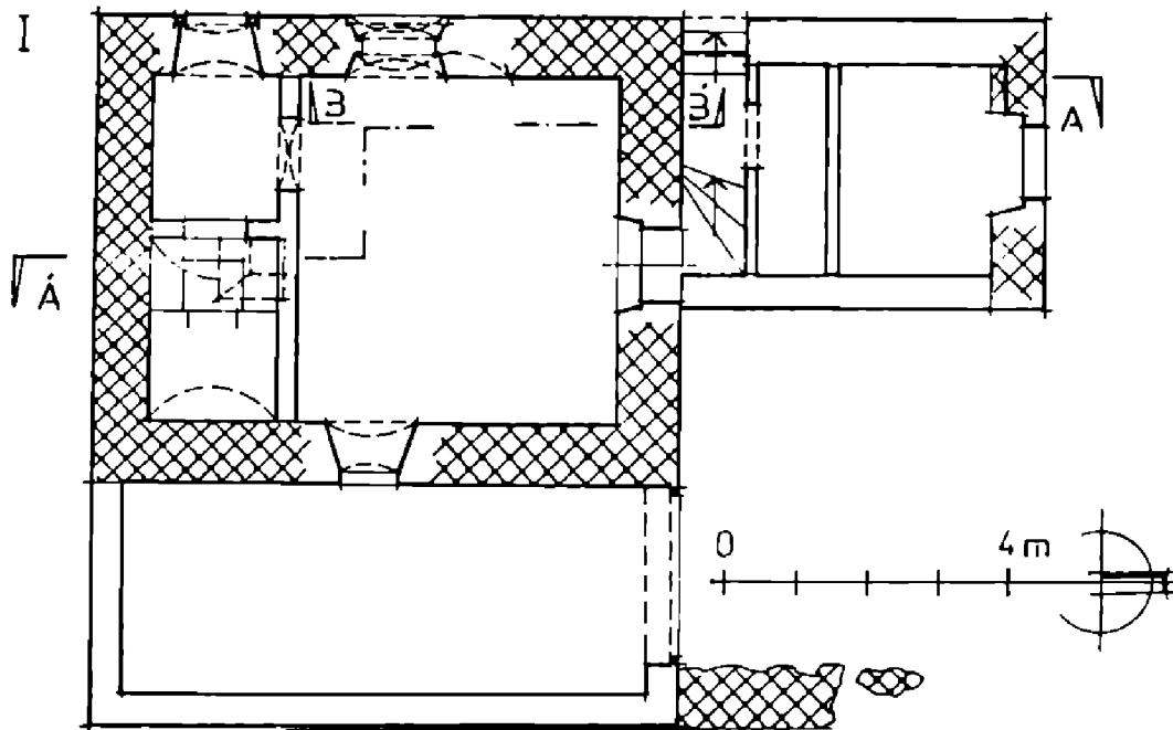
Obr. 14. Vrhavěč, objekty v prostoru bývalé gotické věže. Šrafovane vyznačeno zdívo pravděpodobně středověkého původu. Stav roku 1984 (kresba J. Anderle).
