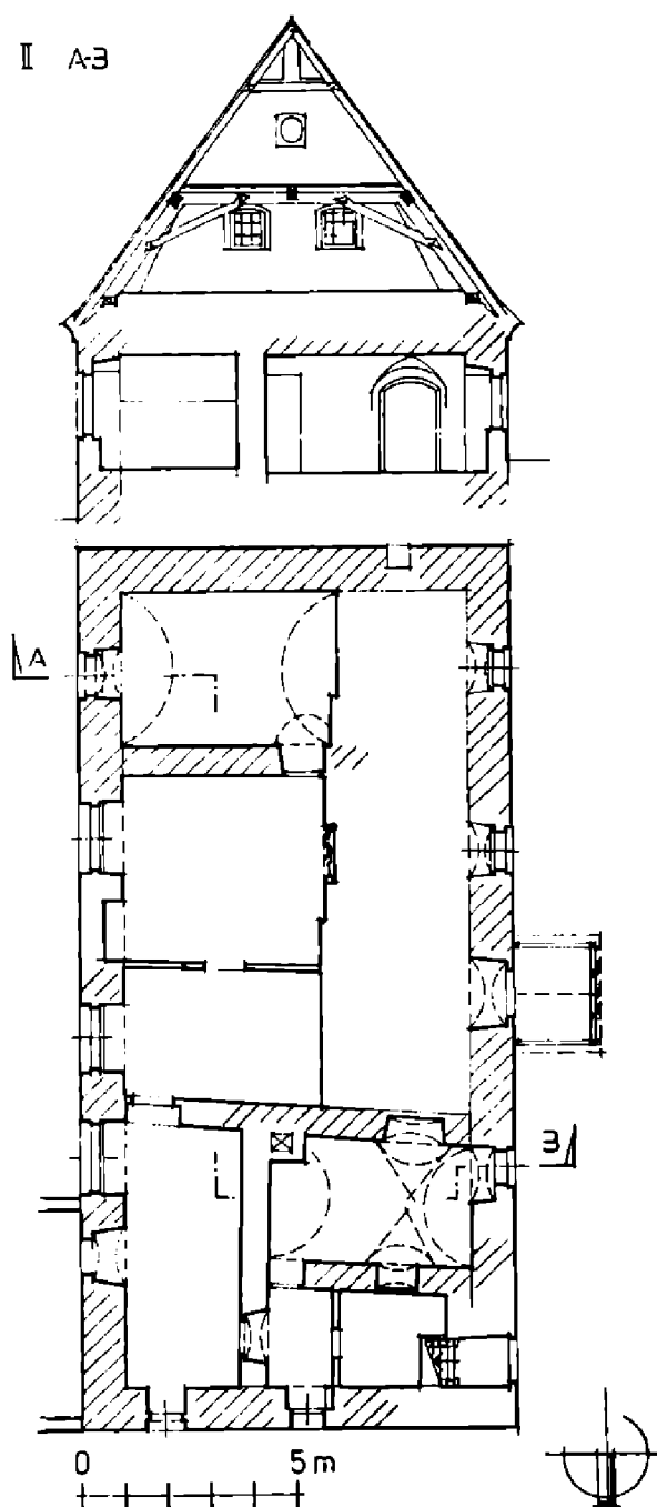
Obr. 12. Vrhavěč, pozůstatek mladší tvrze. Šrafované vyznačeno zdívo pravděpodobně renesanční, stav roku 1984 (kresba J. Anderle).
