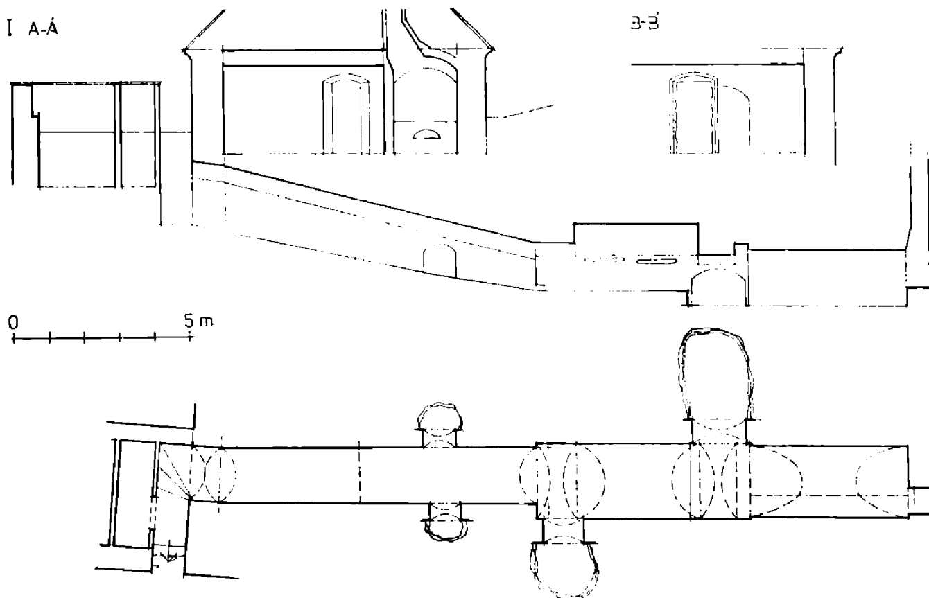
Obr. 16. Vrhavec, objekty v prostoru bývalé věže, řez a půdorys sklepů. Stav roku 1984 (kresba J. Anderle).
