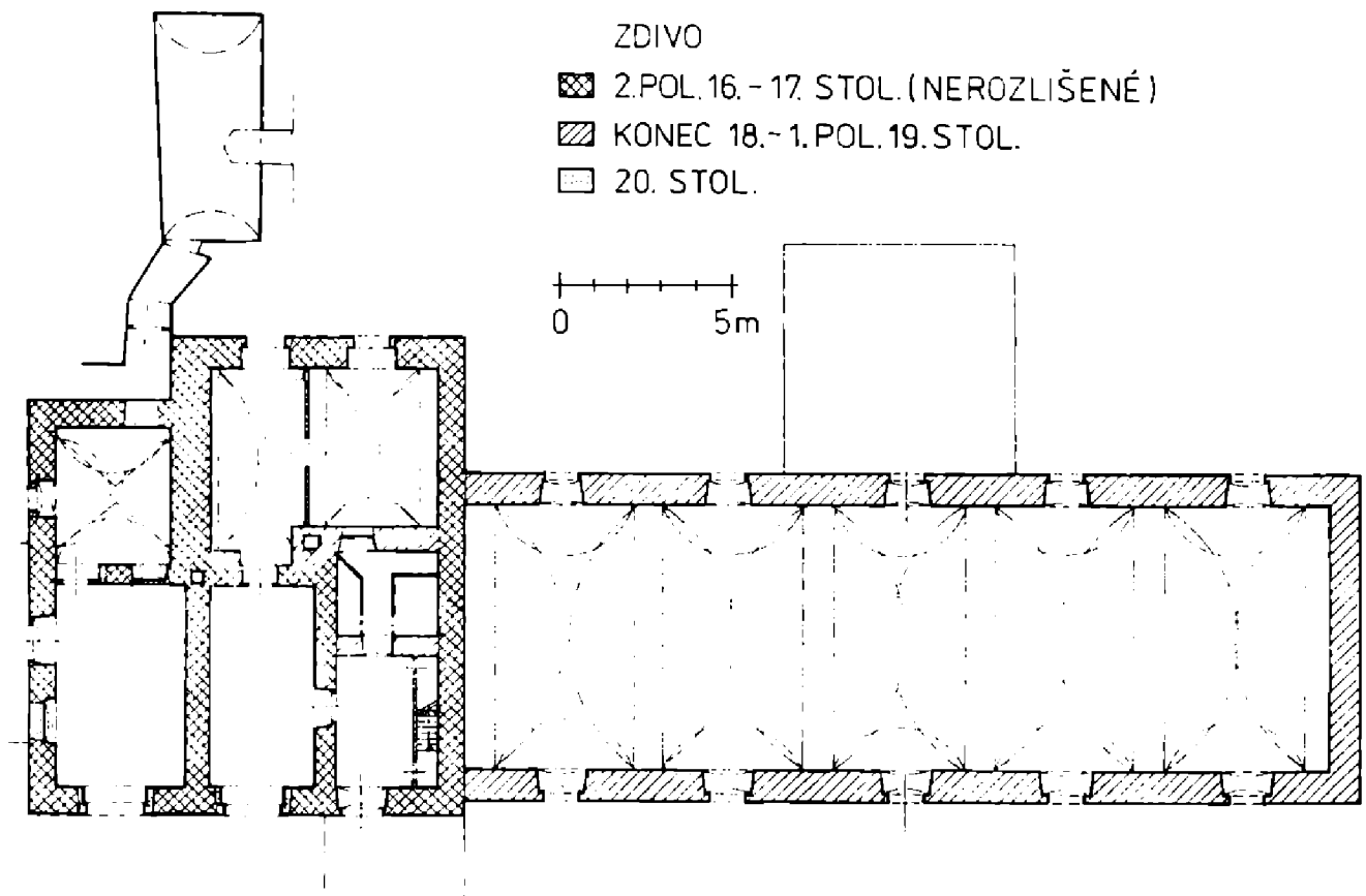
Obr. 7. Kouskova Lhotka, obytné stavení dvora. Zaměření M. Rykl 1986 (ubr. 1-5 a 7 kresba M. Rykl).
