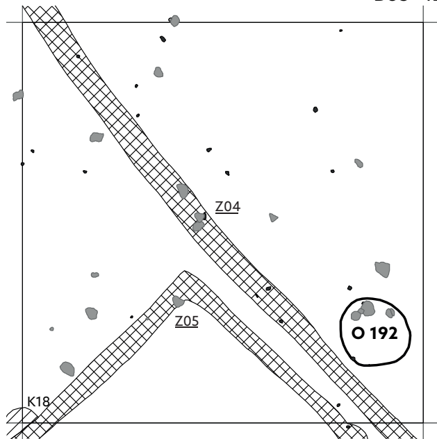
Obr. 154. Plán čtverce B63–42.
