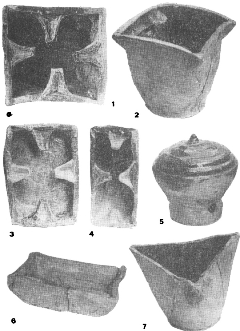
Obr. 4. Liptovská Mara. Ukážka hrncovitých, miskovitých a cibulovitých kachlíc.
