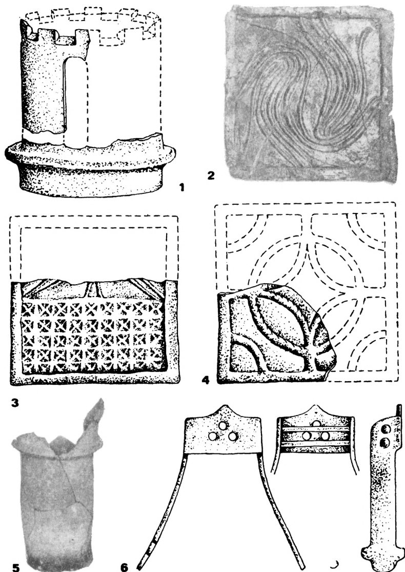
Obr. 3. Liptovská Mara (1-3, 5, 6), Parisovce (4). 1 - vrcholová válcová kachlic, 2-4 - reliéfne zdobené dosky komorových kachlíc, 5 - technický prvok pece, 6 - strmeň z deštrukcie pece.
