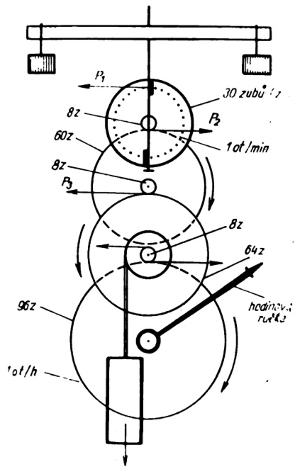
Obr. 6. Schéma přenosu sil v luhýřových hodinách. Podle St. Michala.
