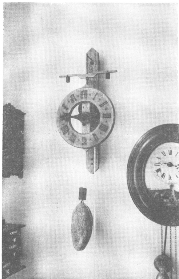
Obr. 1. Švýcarská funkční replika dřevěných hodin z roku 1341.
