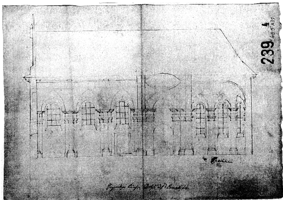
5. Carl Antoni Reina: Řez kostelem Nejsvětější Trojice v Sezemíciích u Pardubic, zachycující navrhované úpravy (kol. 1724, Archiv Pražského hradu, Stará sbírka plánů, sign. 239/3, inv. č. 4230).
