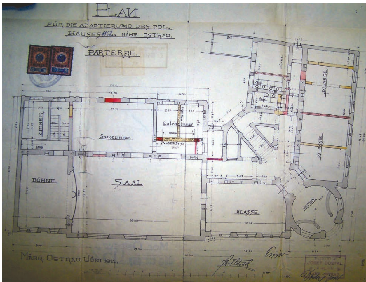
15 – Stanislaw Bandrowski, Josef Dostal, půdorys přizemí Polského domu , 1917. Moravská Ostrava, Archiv Stavebního úřadu Moravská Ostrava a Přívoz, fond dokumentů a plánů pro objekt č. p. 1152
