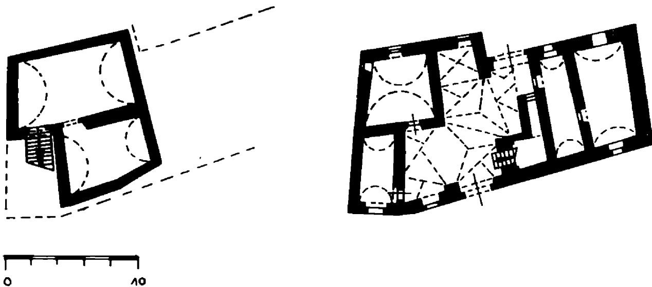
Obr. 2. Tábor, čp. 119. Klokotská ulice. Sklepy a přizemí.
