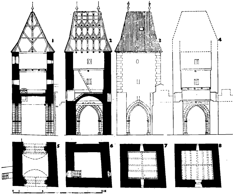
Obr. 6. Pražská brána. 1 – žez s pohledem k západu, 2 – žez s pohledem k severu, 3 – pohled na severní průčelí, 4 – rekonstrukce raně gotického uspořádání interiéru v žezu s pohledem k severu, 5–8 půdorys přízemí a jednotlivých pater, 1–3, 5–8 upraveno podle zaměření z archivu ŠUPPOP Praha, r. 1922. Kresba autor.
