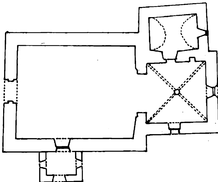
Obr. 1. Kraskovo, půdorys dnešního kostela.
