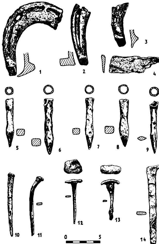
Obr. 3. Hrad Engelsberk (Vizovické vrchy) — soubor železných předmětů.
