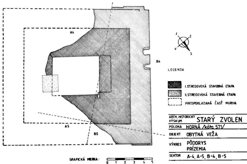
Obr. 4. Starý Zvolen, odkrytá a zameraná časť základov obytné veže komitátneho hradu.
