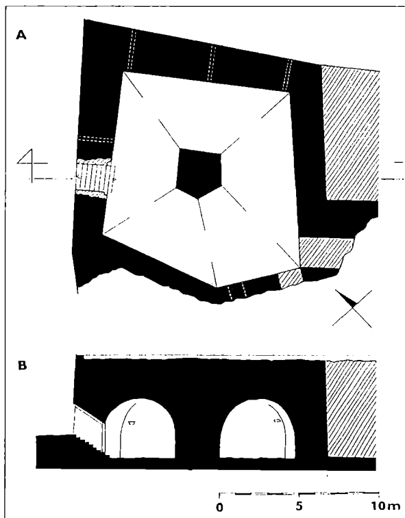
Obr. 14. Nový Světlav – S bastion; A – půdorys (šrafované vyznačen zásyp a mladší zdivo), B – řez (šrafované – zásyp v prostoru kurtíny).
