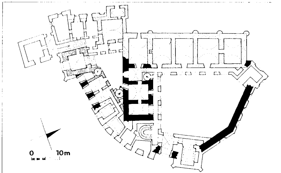
Obr. 6. Nový Světlov – půdorys přízemí jádra s vyznačením předpokládaných stavebních fází: černě – 2. pol. 15. stol., křížem šrafované – po pol. 16. stol., šrafované – 2. půle 16. stol., přetřhávané šrafované – 1. pol. 17. stol., tečkované – 18.– pol. 19. stol., bíle – pol. 19. stol. (kresba R.Vrta).
