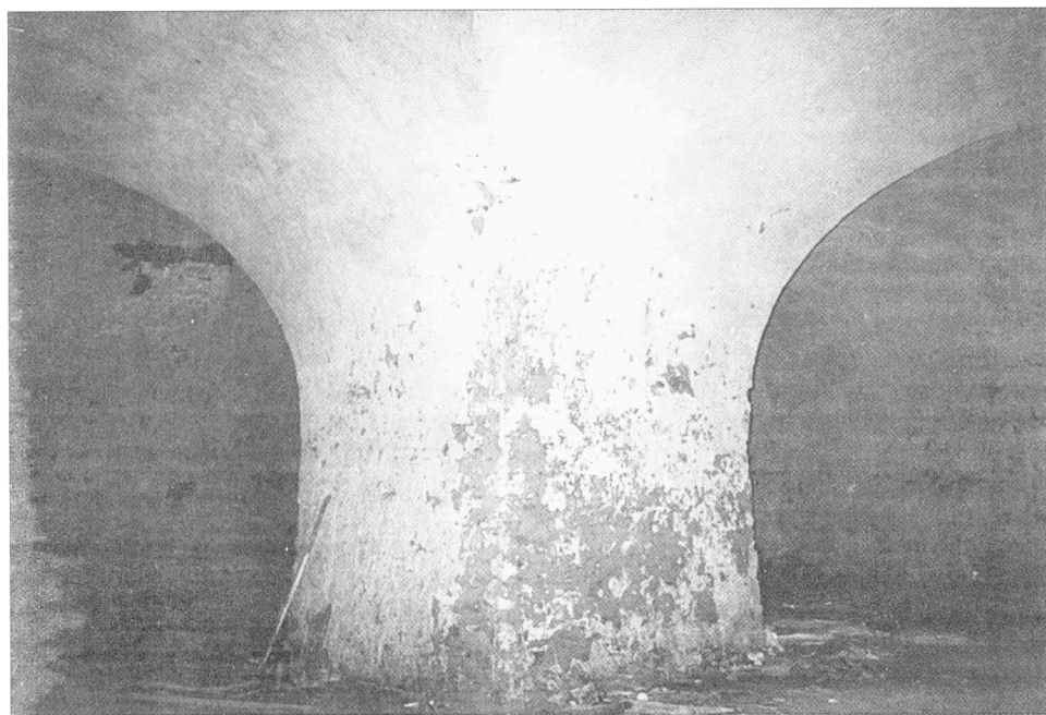
Obr. 15. Nový Světlav – střední pilíř v místnosti S bastionu (foto R.Vrla 2000).
