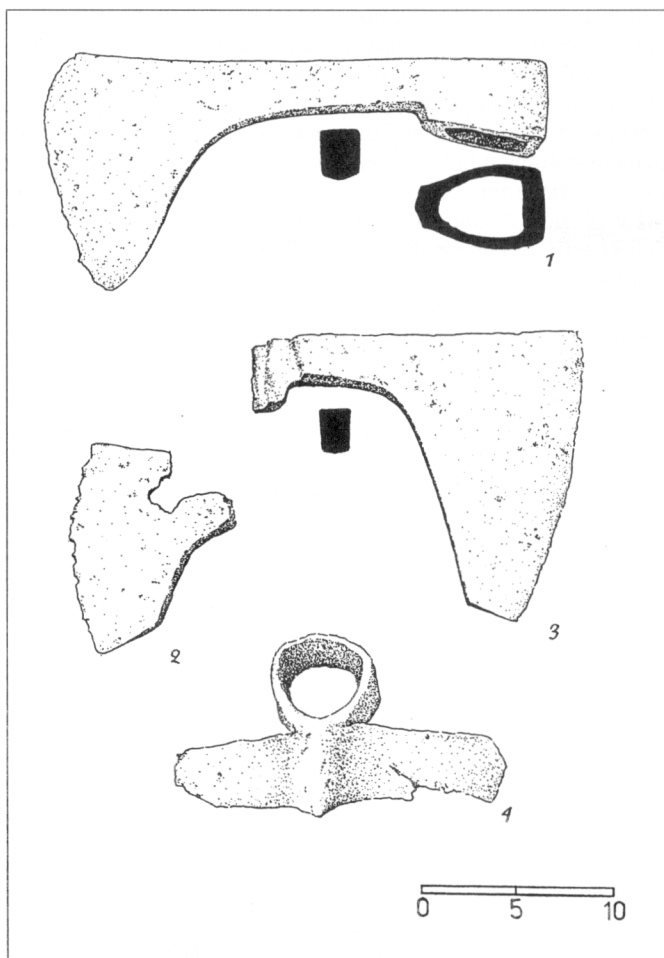
Obr. 9. Čabradský Vrbovok-Táborisko. Kovový inventár z opevnenej polohy. Kreslila M. Severínyová.
