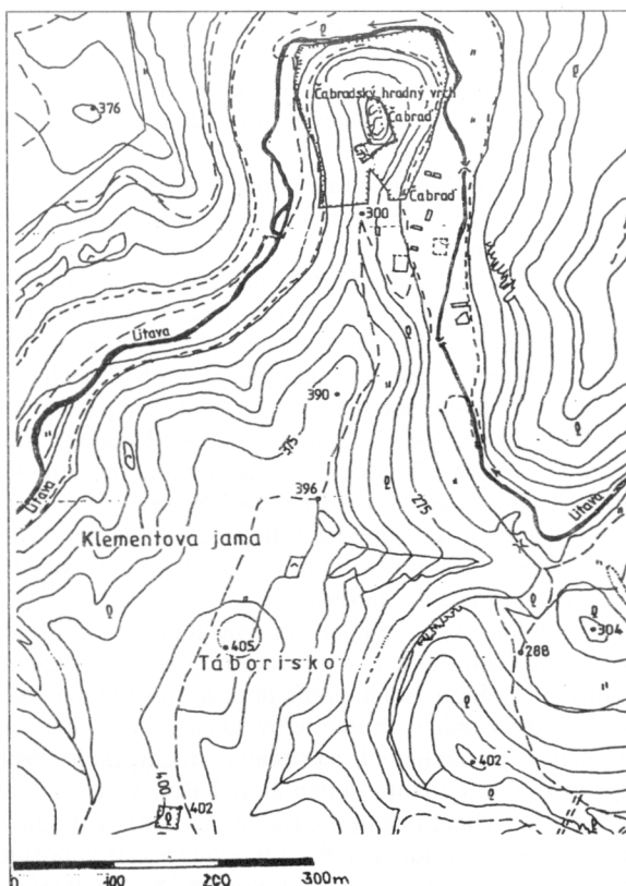
Obr. 1. Hrad Čabrad a archeologická lokalita Táborisko, situačné zameranie.
