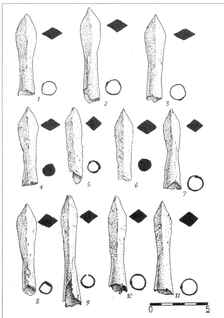
Obr. 8. Čabradský Vrbovok-Táborisko. Hroty striel z opevnenej polohy. Kreslila M. Severínyová.
