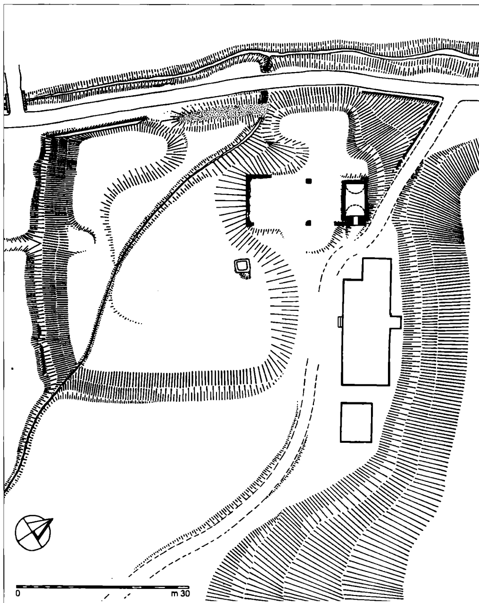
Obr. 1. Ondřejovice, půdorysné zaměření, stav v roce 2005 (Pavel Kouřil–Dalibor Prix).
