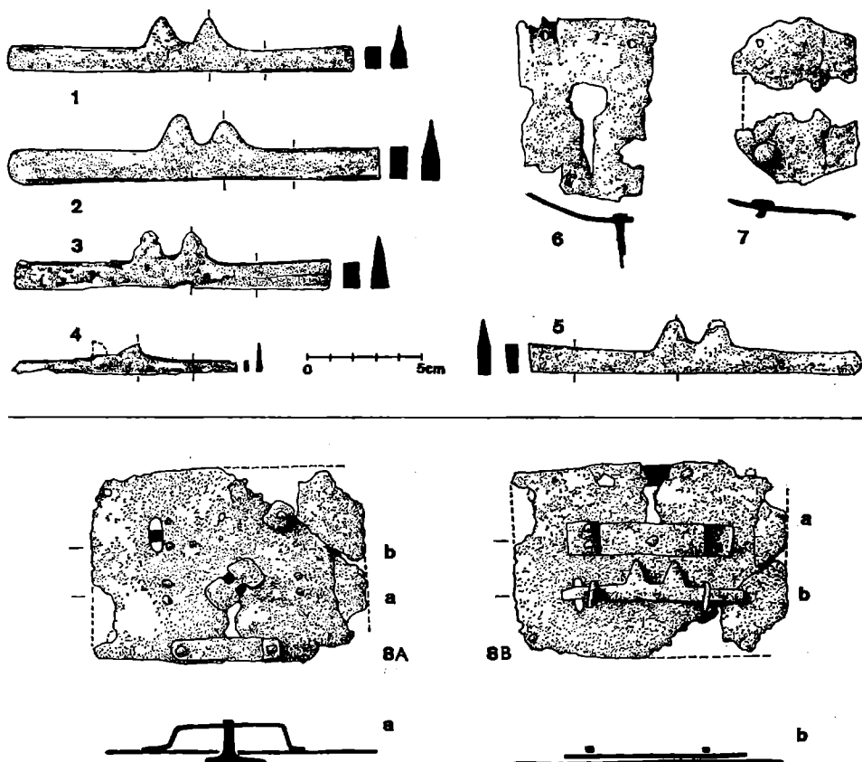
Obr. 3. Břeclav-Pohansko. Železné závory zámků (1—5) a kování klíčových otvorů (6—7). Od obj. 112/VD ve čtv. A 13—75 (1); ze čtv. A 9—53 (2); od obj. 67/LŠ ve čtv. B 69—86 (3); obj. 58/LŠ (4); obj. 168/LŠ (5); sonda 3/SP (6); obj. 55/LŠ (7). — Der Runde Berg bei Urach. Rub a líc zámků s dvouzubou závorou z vrstev 9.—10. stol. na alamanském sídlišti (8a,b — podle U. Kochové).
