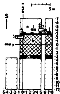
BŘECLAV-POHANSKO Val I. (1961-63) Schema výkopu
