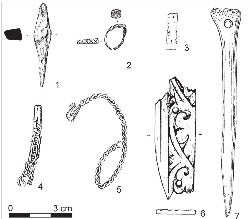
Obr. 12. Brno, Josefská 7. Výběr nekeramických nálezů. 1 – hrot šípů, s. j. 129, přelom 14. a 15. století; 2 – prsten se šitkem, s. j. 119, druhá polovina 13. století; 3 – kování, s. j. 1124, suterén 639, druhá polovina 14. až první polovina 15. století; 4 – zlomek šperku ze spletených drátků, s. j. 281, přelom 12. a 13. století; 5 – záušnice z tordovaného drátu, s. j. 120, druhá čtvrtina 13. století; 6 – kostěné obložení, s. j. 227, druhá čtvrtina až druhá polovina 13. století; 7 – kostěná jehlice únětické kultury z kontaktní vrstvy s. j. 244 mezi jámou 600 a pravěkým objektem č. 601. Předměty č. 2-5 vyrobeny z kovů na bázi mědi. Kresba L. Dvořáková.
