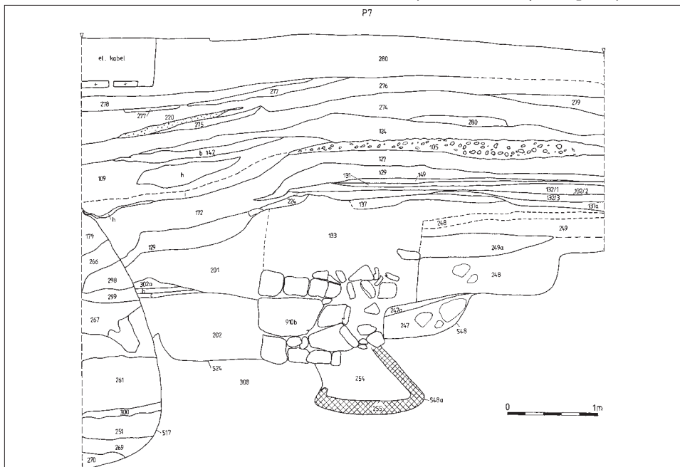
Obr. 13. Josefská 8. Profil při uliční čáře. Jáma 524 ze zdi 910b – pyrotechnologické výrobní zařízení porušující pec v jámě 548–548a, obě z první poloviny 13. století; 131, 132/1–3, 1249, 137, 137a – podlahové úpravy povrchového domu, přelom 13. a 14. století; výše souhrn hlinitých a šterkových vrstev 14. století; 517 – obilnice, 14. století. Archiv Archaia Brno, o. p. s., Procházka 1996.
