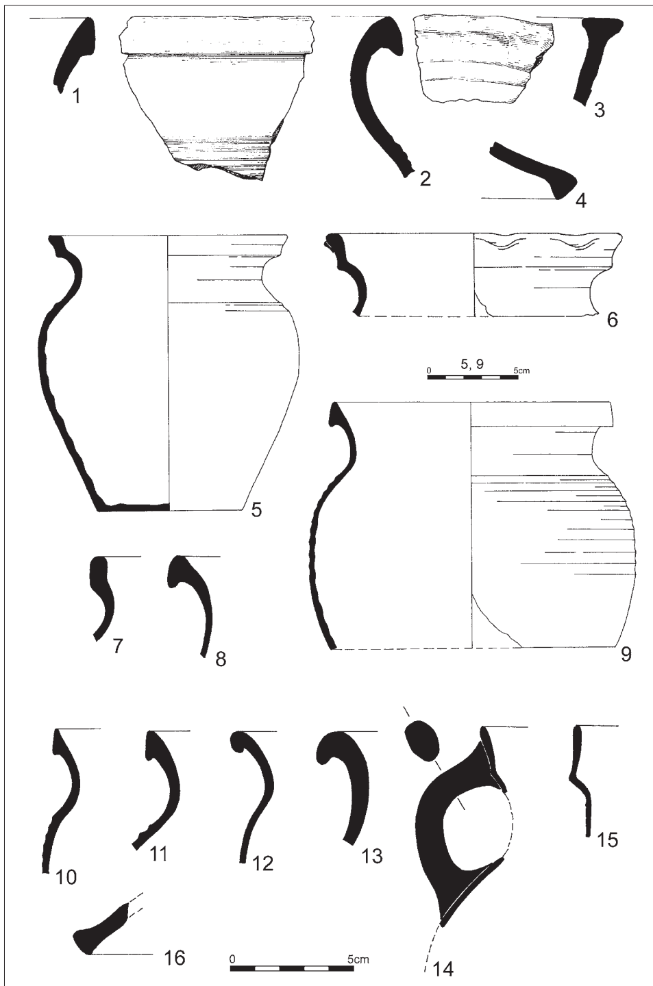
Obr. 10. Brno, Josefská 7. Keramika z přelomu 14. a 15. století. Jímka 692, s. j. 1386. Kresba L. Dvořáková (1–4) a Š. Trávníčková (5–16).
