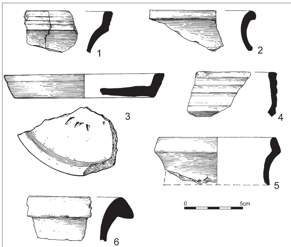
Obr. 9. Brno, Josefská 7. Keramika závěru 13. a první poloviny 14. století. 1–6 – s. j. 229. Kresba L. Dvořáková.
