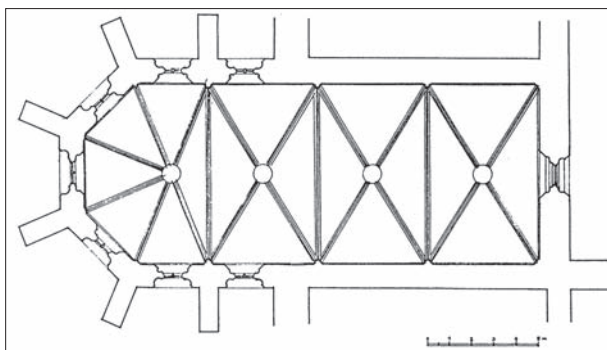
Obr. 5. Zvolen, zámok, pôdorys prízemnia kaplnky. Podľa Matuščák 2000, obr. 3.
