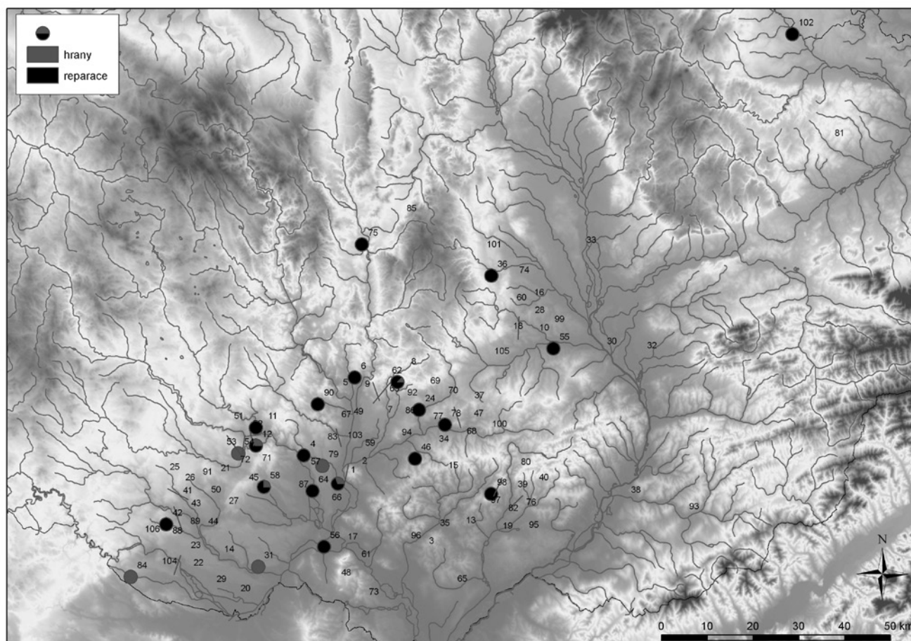
Obr. 137: Distribuce hran jádra a reparačních úštěpů ve starší době bronzové. Na mapový podklad vložila J. Mazáčeková.
