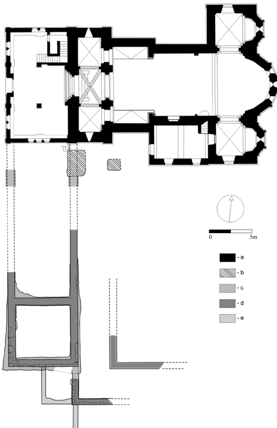
Obr. 26. Biňa, niekdajší kláštorňý kostol premonštrátov a archeologicky preskúmané zvyšky vnútornej klauzúry. a – stojaci kostol, b – najstaršie, archeologicky zistené murivá, c – základy, d – nadzákladové časti murív, e – prístavby. Podľa Pomfyová–Samuel–Žažová 2014 na základe nepublikovaných archívnych materiálov A. Habovštiaka.
