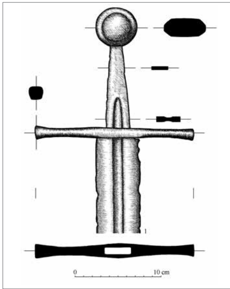
Obr. 5. Meč z obce Bohdan. Prekreslenie základných konštrukčno-morfologických častí rukováti meča. Kresba Igor Prokhenko.
