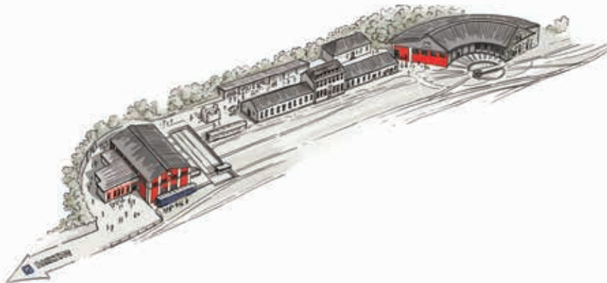
Abb. 4: Die Abbildung zeigt die Anlage des Südbahnmuseums Mürrzuschlag: links die als „Innenraum-Museum“ genutzte „Neue Montierung“ mit der seitlich vorgelagerten Schiebep Bühne, rechts das Rundheizhaus mit vorgelagerter Balancedrehscheibe, in der Mitte das Verwaltungsgebäude der aktuell noch von den ÖBB (Österreichische Bundesbahnen) betriebenen sogenannten „Traktion“; davor Geleise, die zusammen mit der Balancedrehscheibe als Zufahrt für Lokomotivshows, Sonderfahrten sowie -veranstaltungen des „SÜDBAHN Museum Mürrzuschlag“ genutzt werden. Bildnachweis: SÜDBAHN Museum Mürrzuschlag
