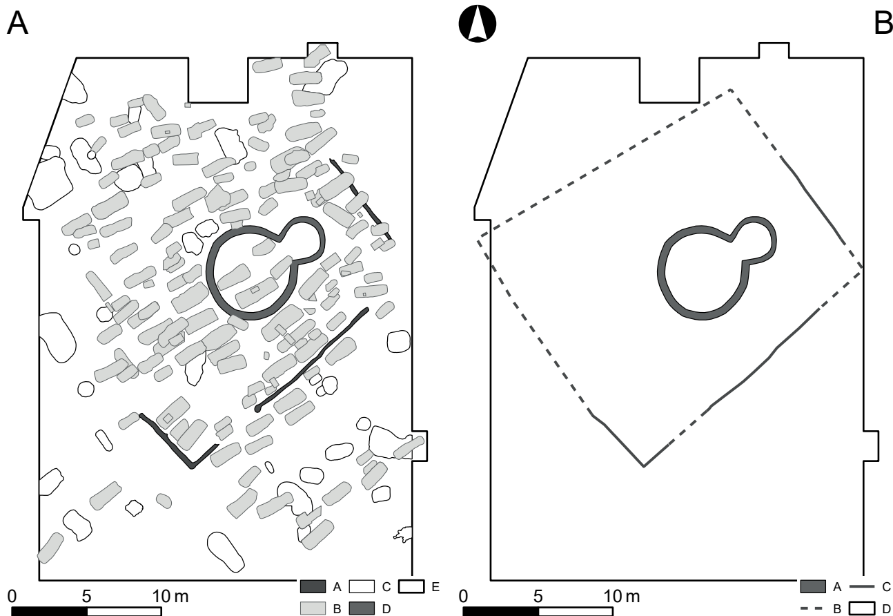
Obr. 8. Břeclav – Pohansko, Severovýchodní předhradí. A) Celkový plán pohřebiště se zachycenými žlábkami. Legenda: A – žlábek ohrazení, B – hroby, C – objekty, D – základy kostela, E – prozkoumaná plocha; B) idealizovaný pravděpodobný průběh ohrazení areálu. Legenda: A – základy kostela, B – předpokládaný průběh ohrazení, C – dochované žlábkové ohrazení, D – prozkoumaná plocha.
