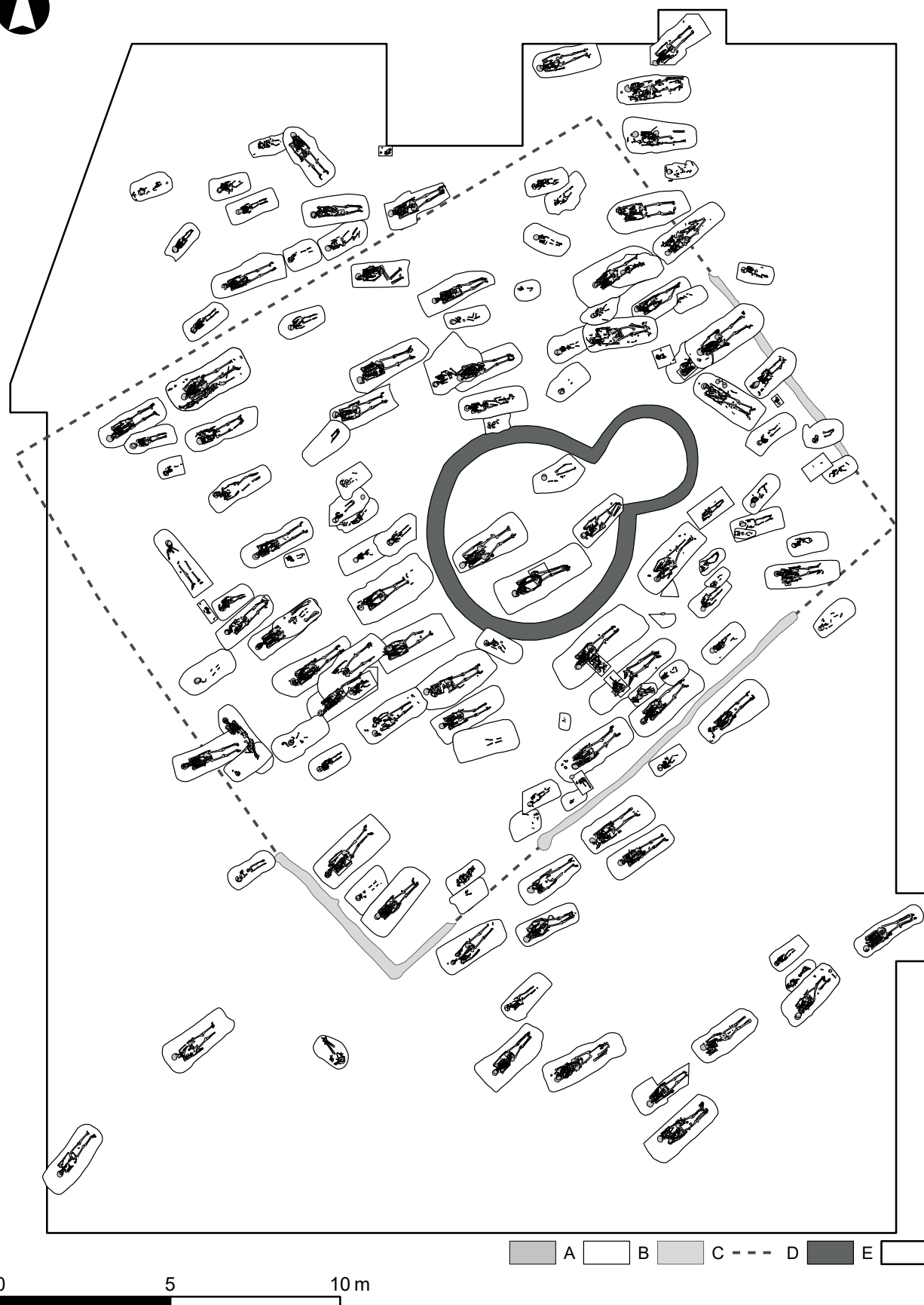
Obr. 7. Břeclav – Pohansko, Severovýchodní předhradí. Celkový plán pohřebiště u druhého kostela. Legenda: A – lidské kosti, B – hrobová jáma, C – žlábek po ohrazení, D – předpokládaný průběh ohrady, E – základy kostela, F – prozkoumaná plocha.
