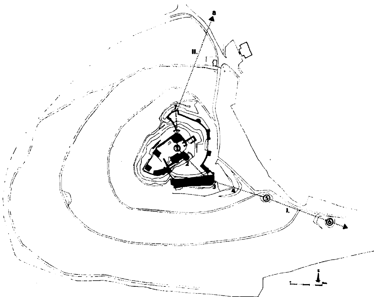
Obr. 8. Státní hrad Klenová — schéma předpokládaného opevnění. I. Jihovýchodní rameno: 1 předpokládaná válcová věž, 2 — půlválcová bašta, 3 — bašta v nároží dnešního zámku, 4 — val, 5, 6 — předpokl. místa předsunutých obranných objektů; II. Severní rameno: 7 — severní bašta, 8 — předpokl. obranný objekt v místech dnešní kaple sv. Felixe (F. Kašíčka).
