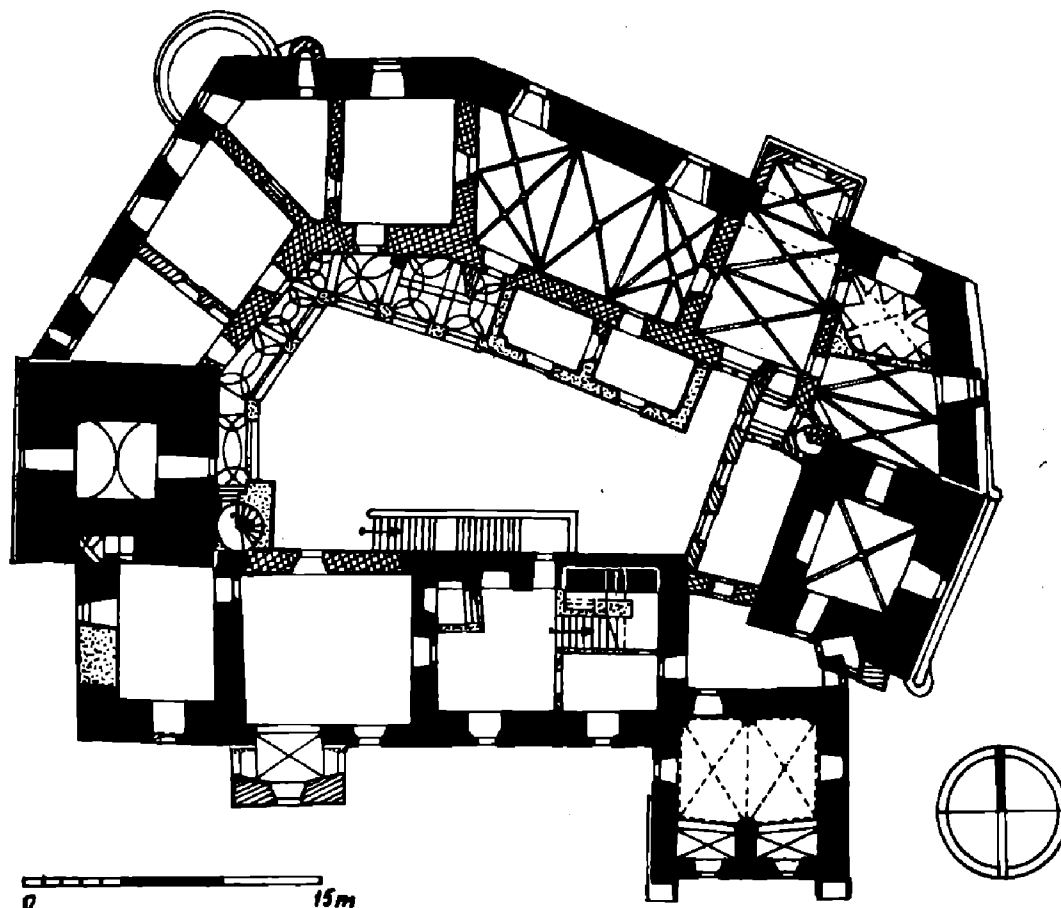
Obr. 10. Buchlov, okr. Uh. Hradiště. Půdorysné členění nejstaršího jádra hradu: plně zdivo 2. pol. 13. stol., mřížkovně zdivo 14. stol., šrafovaně zdivo 15.–16. stol., tečkovaně zdivo 17.–18. stol. Příklad podunajské dispozice s hranolovými věžemi (podle A. Bartuška–K. Svobody 1956).
