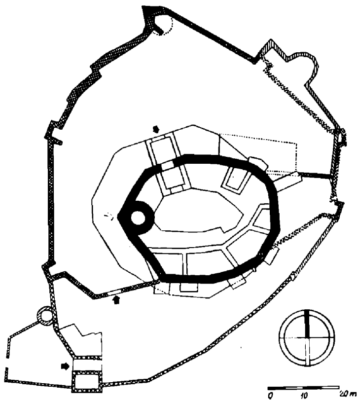
Obr. 13. Boskovice, okr. Blansko. Schéma vývoje hradního půdorysu; plně vyznačeno předpokládané jádro ze 13. stol., hustší mřížky – hradební okruh z 15. stol., řidší mřížky – rozšíření půdorysu hradu kol. roku 1500. šikmo šrafovány renesanční zásahy. Příklad hradu s obvodovou zástavbou a věží s břitem (podle F. Kašíčky 1973).
