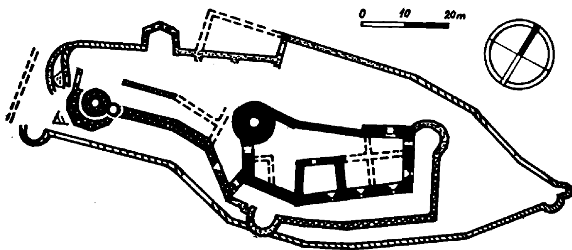
Obr. 16. Nový Cimburk, okr. Kroměříž. Půdorys hradu; plně nejstarší část do pol. 14. stol. se zrněně vyznačeným opevněným přístupem k jádru hradu, mřížkovane zdívo z doby kol. pol. 15. stol., šrafované zdívo z konce 15. stol. a tečkované z 1. pol. 16. stol. Příklad bergfritové dispozice s fortifikací mající zamezit přístup k hradnímu jádru (podle D. Antořové 1966).
