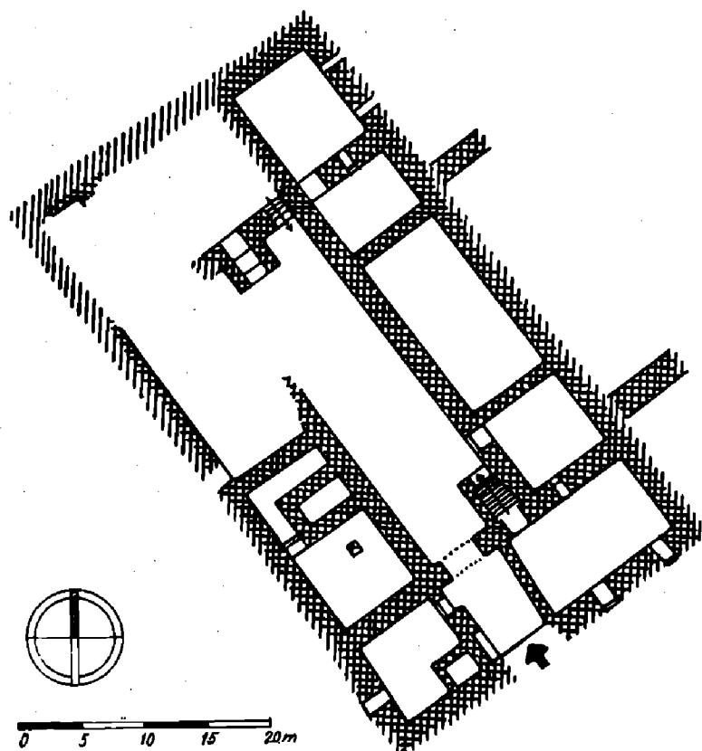
Obr. 18. Melice, okr. Vyškov. Půdorys hradu; mřížkovně vyznačeno zjištěné zdivo, šrafované předpokládaný průběh archeologicky nezkoumaných základů hradu. Příklad dispozice vycházející z dvoupalácového typu (podle J. Zháněla 1967a).
