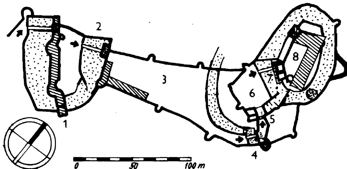
Obr. 19. Helištejn, okr. Přerov. Schematizovaná skica půdorysu hradu s vyznačením nejdůležitějších částí (1 – první příkop se štítovou zdí a první bránou, 2 – druhý příkop a druhá brána, 3 – druhý dvůr, 4 – třetí příkop a třetí brána, 5 – čtvrtá brána, 6 – třetí dvůr – tzv. Kravašské předhradí, 7 – čtvrtý příkop a pátá brána, 8 – původní jádro hradu posl. čtvrtiny 13. stol. se šrafovaně vyznačeným půdorysem renesanční přestavby paláce). Příklad rozsáhlé dispozice 15. stol. s rozlehlým předhradím a postupně rozšiřovanými předsunutými fortifikacemi (podle Z. Gardavského 1959).
