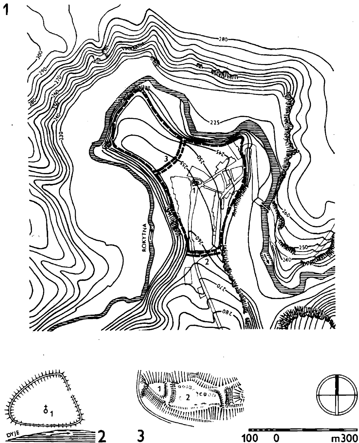
Obr. 4. Fortifikace 11.–12. stol. 1 – Rokytná, okr. Znojmo (1 – pozdněrománský kostel, 2 – vnější příkop, 3 – vnitřní příkop); čárkovane vyznačen předpokládaný průběh opevnění), 2 – Dol. Věstonice, „Vysoká zahrada“, okr. Břeclav (1 – poloha kostela; upraveno podle J. Poulika 1948–1950), 3 – Radkov, okr. Svitavy (1 – hrad, 2 – předhradí; podle J. Mackerleho 1957a).
