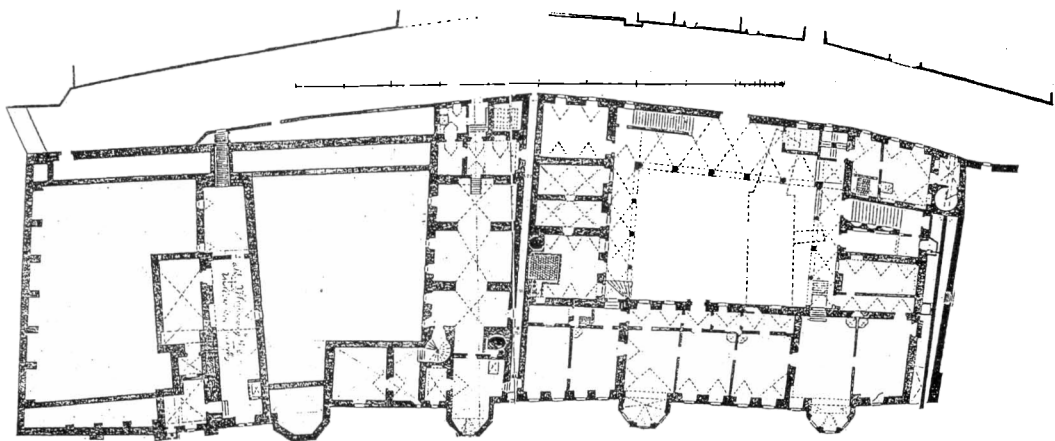
Obr. 6. Pražský hrad – Púdorys přízemí Rožmberského paláce se sklepy pod bývalou Švaberskou částí r. 1738 (APH 125/10).
