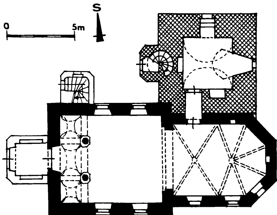
Obr. 4. Vrbeno u Mělníka – příklad pozdně gotické přístavby věže k vesnickému kostelu, která plnila funkci zvonice a útočiště. Kresby F. Kašíčka.
