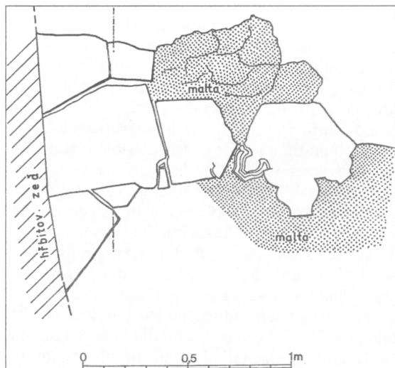
Obr. 3. Detail základů třídlňné hruškovité přípory na severní straně polygonálního závěru.
