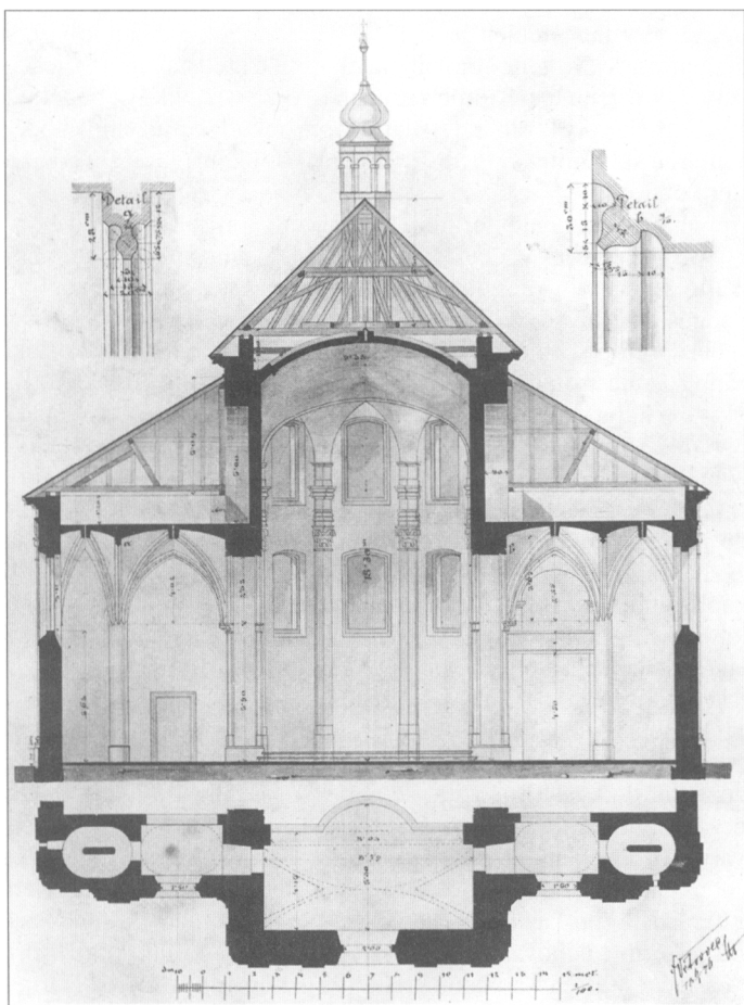
Obr. 8. Příčný řez kostelem sv. Petra a Pavla před novogotickou přestavbou se zakreslenými gotickými profily žebér a s barokní podsíní z r. 1729. Zaměřil J. Větrovec 1876 (sign.). Vyšehrad kapitulní farní úřad, sbírka plánů (nesign.). Foto O. Hilmerová.
