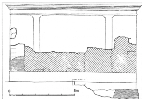
Obr. 6. Štůpa, hřbitovní kaple – zaměření V zdi kaple s hrubou analýzou stáří líců zdiva, odkrytého při sejmutí spodní části novodobých omítek (rozhraní odstraněné omítky vyznačeno silnou čarou): vodorovně šrafované – lomové gotické zdivo, šikmo šrafované – pozdější, či později upravované líce zdiva. Na levém nároží zbytky gotické exteriérové omítky s rytými linkami kvádrování, omítky i blok zdiva ukončen vpravo svislou spárou, indikující nasazení asanovaného presbytáře (kresba: R. Vrla 2002).
