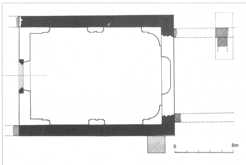
Obr. 4. Štípa, hřbitovní kaple – půdorys se zjednodušenou analýzou stáří zdiva: černě – stojící středověké zdivo (nejdou zde zaznačeny pozdější průrazy a niky, černě je vyznačeno i kamenné ostění středověkého portálu, umístěné dnes v druhotné poloze), křížem šrafované – středověké zdivo odhalené archeologickou sondáží (datace příčky v presbytáři je nejistá), šrafované – základ pilíře při JV nároží lodi, bíle – pozdější úpravy.
