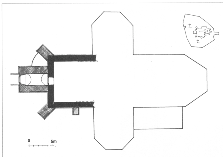
Obr. 11. Brumov, farní kostel sv. Václava – půdorys kostela s se zjednodušeným vyznačením středověkých a mladších konstrukcí (černě – stojící zdivo kostelní lodi, křížem šrafované – věž a diagonální opěrné pilíře, šrafované – mladší opěrný pilíř, ostatní konstrukce z 19. století; čárkováně naznačena poloha fragmentů interiérové omítky v půdním prostoru) a náčrt situace z mapy stabilního katastru z 20. let 19. století (kresba: Mgr. Eva Staňková a R. Vrla 2002).
