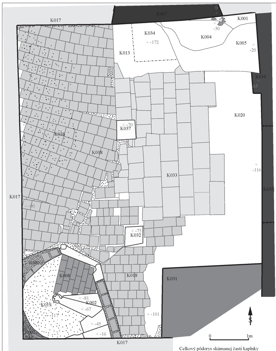
Obr. 2. Celkový pôdorys skúmanej časti kaplnky so zachovanými historickými konštrukciami. Kresba M. Miño.
