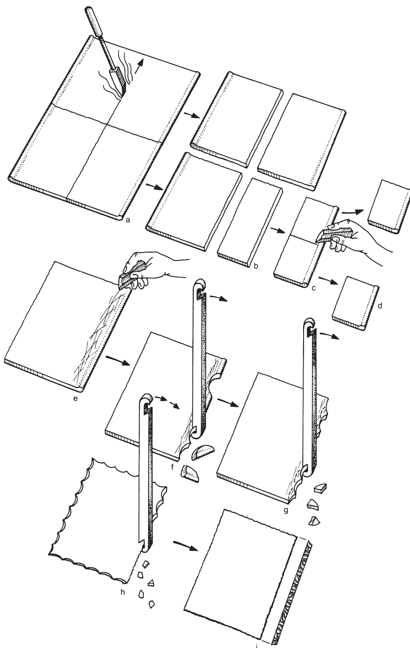
Obr. 9: Rekonstrukce postupu výroby okenních tabulek (podle Kaufmann 2010, abb. 54).
