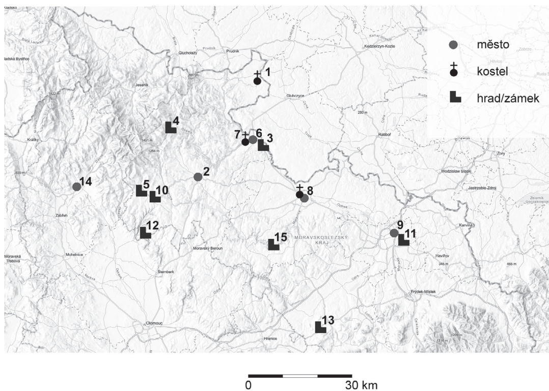
Obr. 4: Lokality s nálezy středověkého a raně novověkého okenního skla v českém Slezsku a na severní Moravě.
