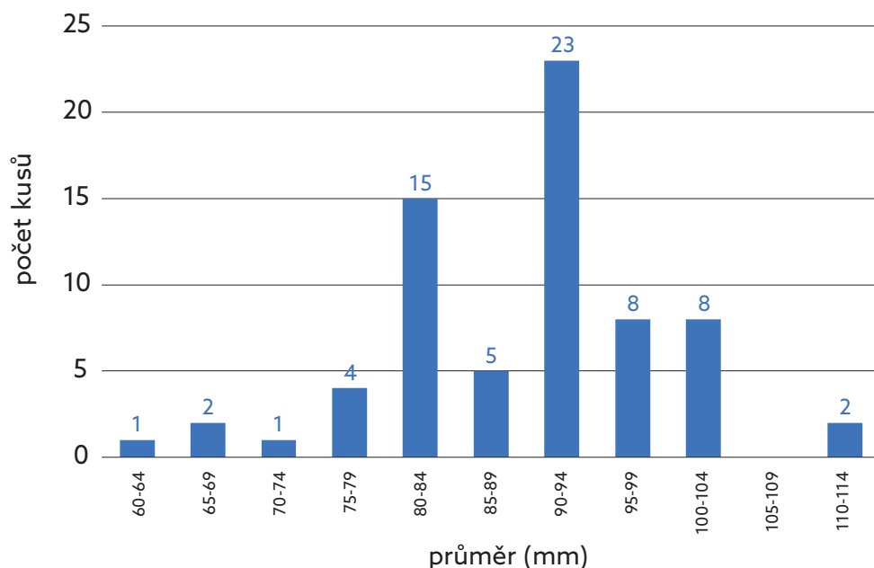
Graf 2: Průměr okrajů lamp z dominikánského kláštera
