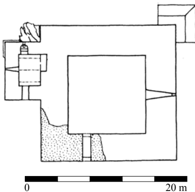
Obr. 1. Přímida, půdorys přízemí donjonu podle Menclová 1972, 1, 104. Tečkované je vyznačeno novodobé doplnění zdíva.
