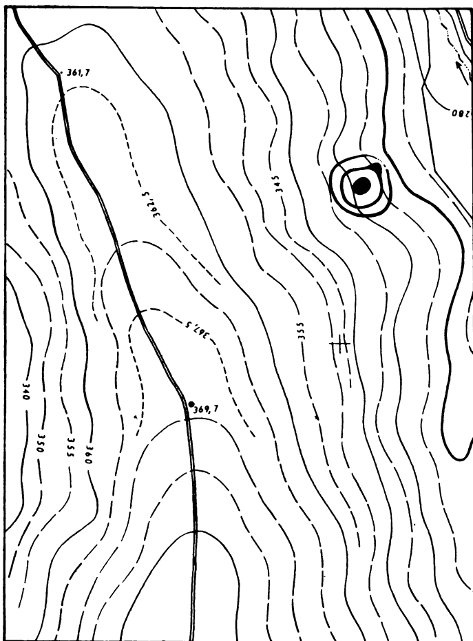
Obr. 1. Hrádek Kepkov – vrstevnicový pláněk.
