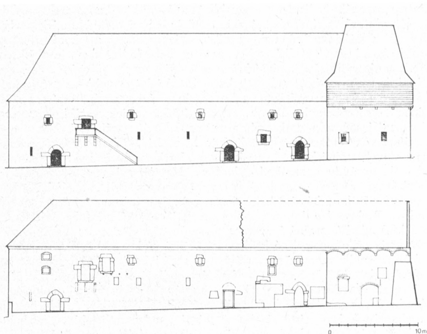
Obr. 8. Tuchoraz (o. Kolín) – Jižní průčelí pozdně gotické hospodářské budovy. Dole současný stav vzniklý mladšími přestavbami, nahoře pokus o rekonstrukci (P. Chotěbor).
