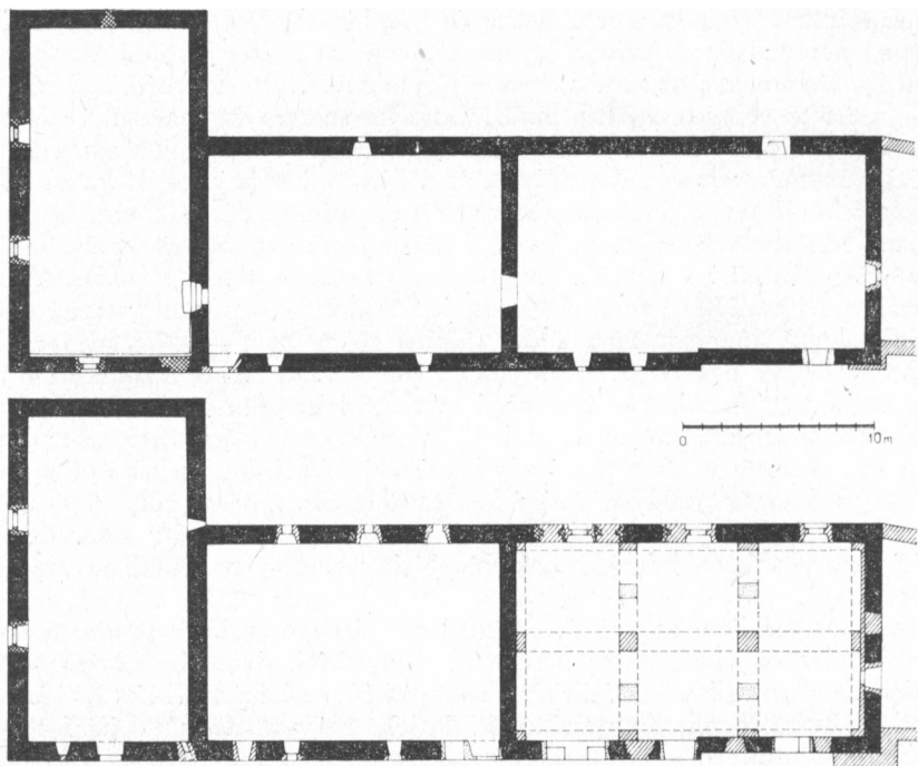
Obr. 7. Tuchoraz (o. Kolín) – Pozdně gotická hospodářská budova v předpolí tvrze. Dole půdorys přízemí, nahoře půdorys patra.
