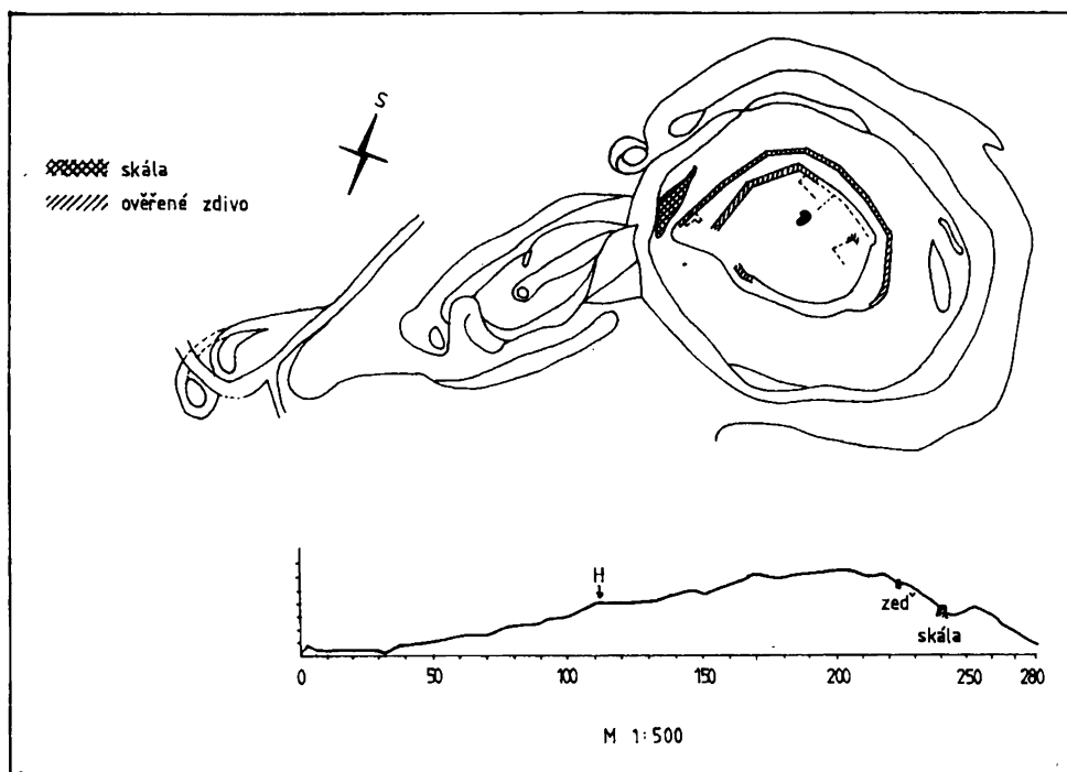
Plán 3. Celkový plán hradu Starého Světlava.
