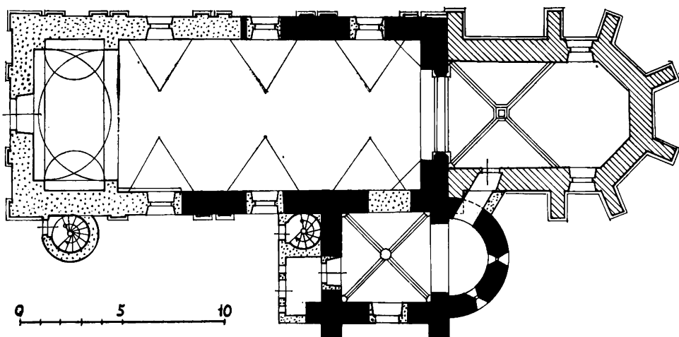
Obr. 1. Půdorys kostela. Povýšení sv. Kříže v Trstěnici u Znojma. Černá – zdívo 13. stol., šrafovaná – gotika, tečkovaná – 16.–19. stol.
