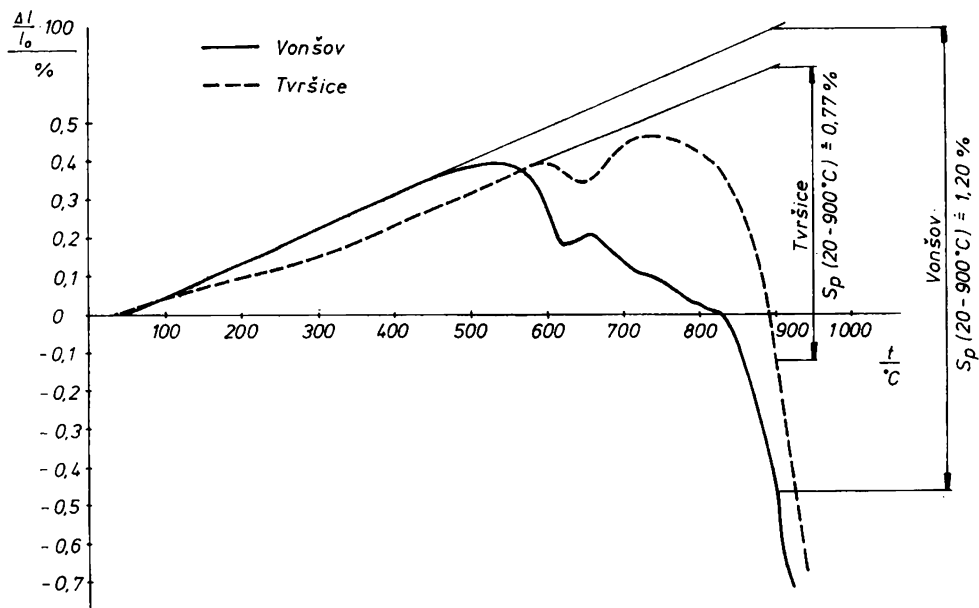
Obr. 1. Křivky DZ čistých jíllů Vonšov a Tvršice s orientačním vyhodnocením smrštění pálením ( S_p ) při výpalu na 900 °C.
