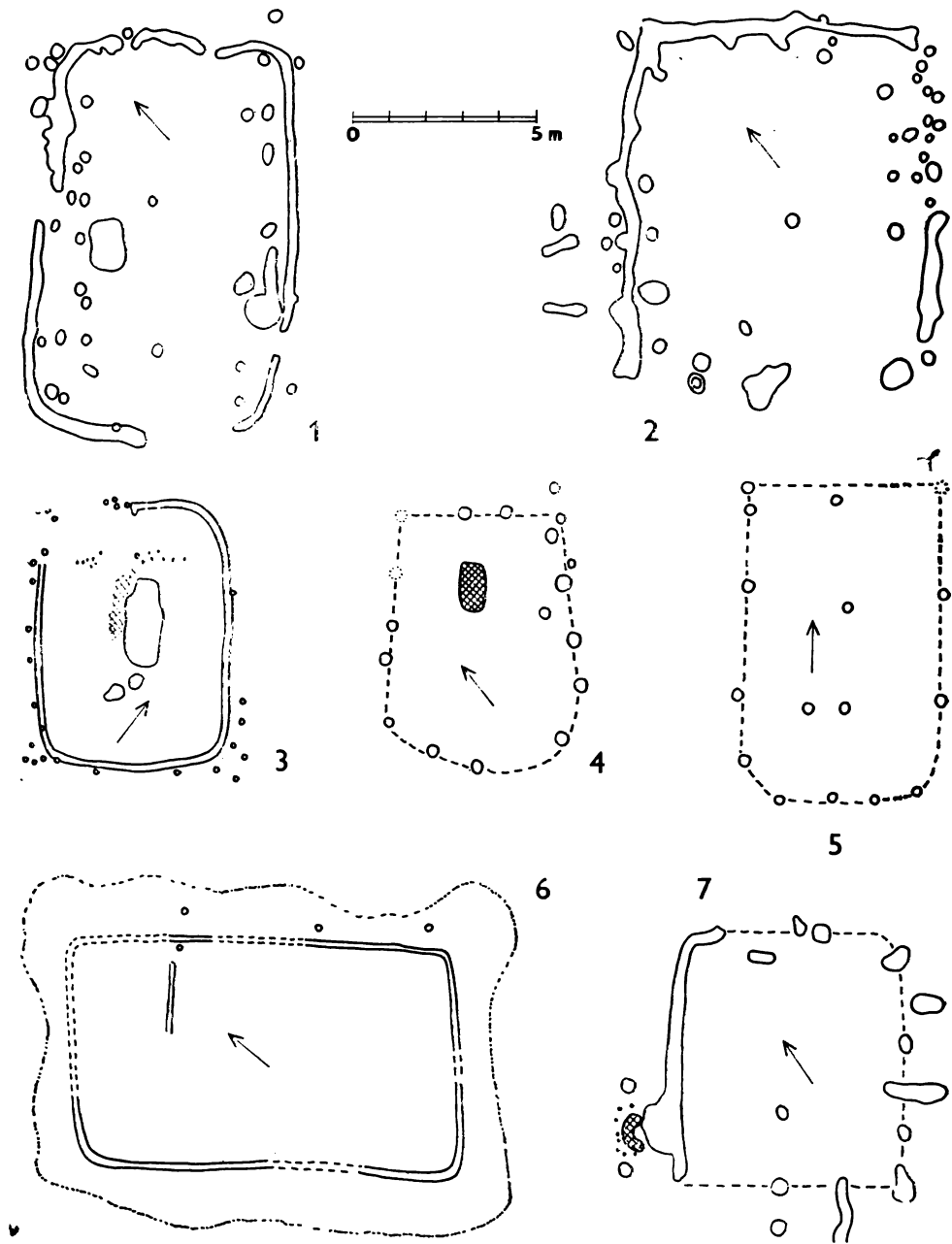
Obr. 9. Velké stavby kúlové konstrukce z velkomoravských hradišť Mikulčic (3) a Břeclavi-Pohanska (1-2, 4-7). Stavby s pletenými stěnami a vnitřním opěrným systémem střešy (1, 2); stavby s pletenými stěnami a vnějším opěrným systémem střešy (3, 6); stavby vymezené kúlovými jamami (4, 5); povrcho- vá stavba s pletenými stěnami a s vysunutým otopným zařízením (7). Tečky na obvodu obr. 6 ozna- čují okraje destrukce propálené mazanice z výpletu stěn. Podle B. Dostála a B. Kavánové.
