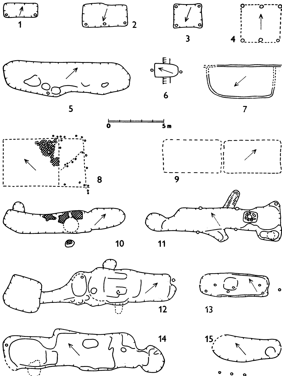
Obr. 11. Hospodářské a dílenské stavby z předvelkomoravského (9) a velkomoravského období (1–8, 10 až 15): kletě (1–4), chlévy a ohrada pro dobytek (5–7), půdorysné schéma kovárny (8) a zlatnické dílny (9) a velké zahlaubené dílenské stavby (10–15). Naleziště: Staré Město, obj. 18/I (1), 13/I (2), 16/I (3), 114/I (6); Sady-Dolní Kotvice, obj. 37 (4); Břeclav-Pohansko, obj. 88/VD (5), 68/2P (7), 106/LS (10), 125/LS (11), 18-49-38/LS (12), 93/LS (13), 103-107-108/LS (14), 105/LS (15). Podle V. Hrubého, Z. Klaníky, B. Klímy, B. Dostála.
