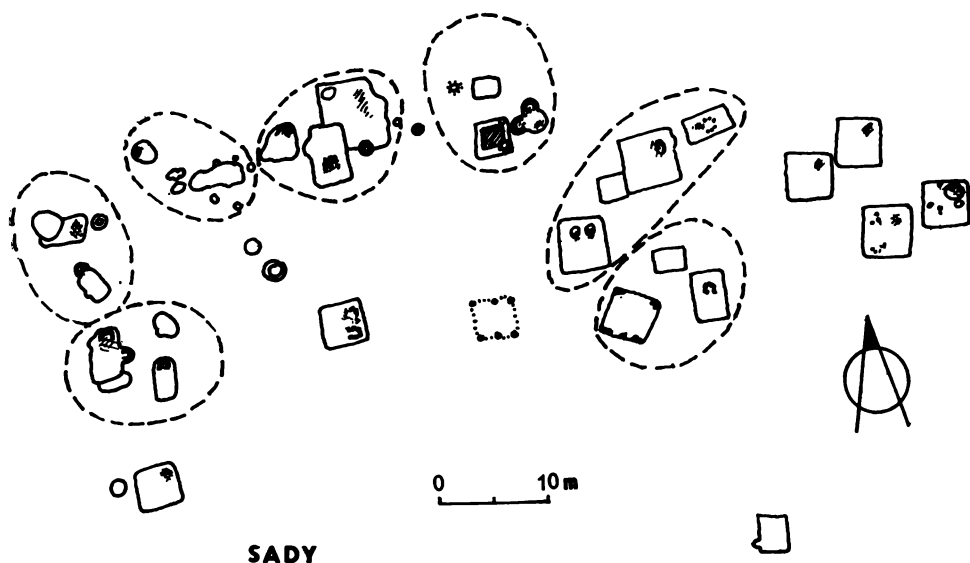
Obr. 4. Půdorysná dispozice velkomoravské osady v Uherském Hradišti-Sadech, trať Dolní Kotvice (zjednodušeně podle K. Marešové). Čárkované označeny jednotlivé dvory.
