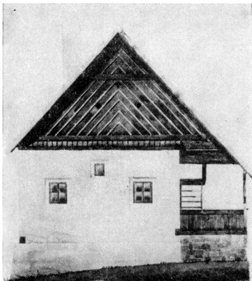
Obr. 5. Rekonstrukce štítového průčelí domu čp. 22 z Živohoště (okr. Benešov), jehož obytnou část tvořila roubená jizba s povalovým stropem, podepřeným jedním hraněným stropním trámem (s datováním 1617), v čelní stěně s jedním horním větracím otvorem. Na vnějšku roubené konstrukce byla hliněná omazávka. Reprodukce dokumentace arch. B. Fialové, archiv SÚPPOP Praha.
