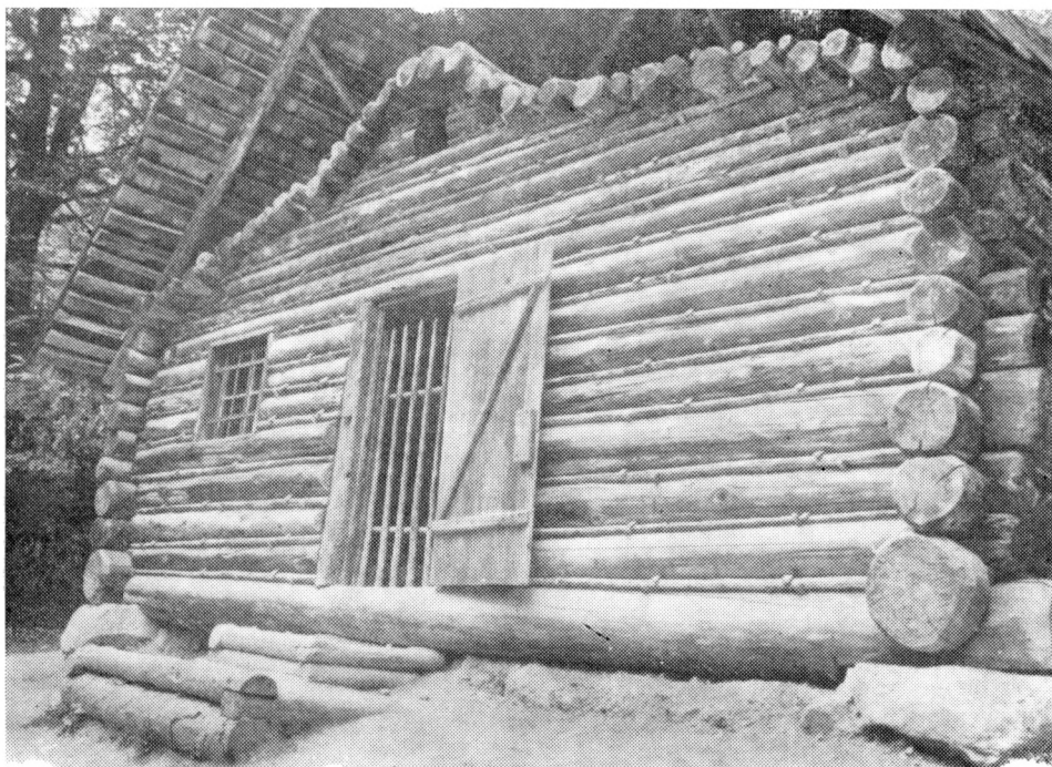
Obr. 8. Skanzen ve Stübingu u Grazu, Rakousko, sezónní jizba dřevařských dělníků, vytápěná ohništěm. Povalový strop je proveden do profilu vlnovkové klenby s dymným otvorem ve vrcholu čelní stěny.
