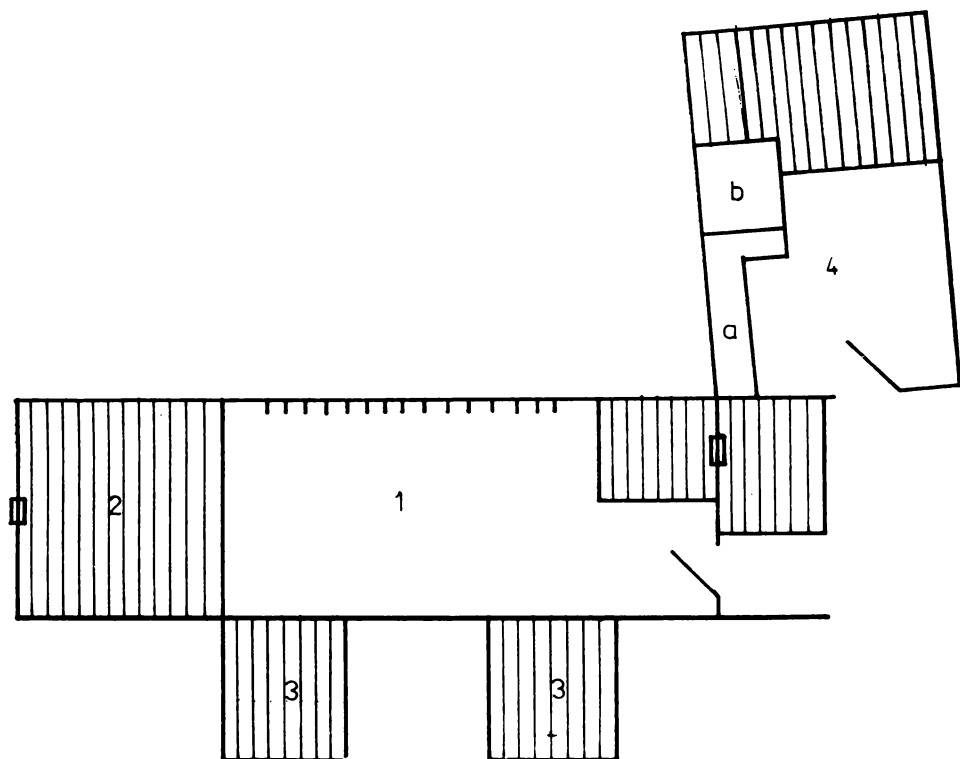
Obr. 9. Božurica, Bulharsko. Zemnicové obydlie rozšírenej rodiny Andrejevovcov. 1 — zemnik, 2 — breg, 3 — bordel, 4 — kufnja, a — ožište, b — pešt. J. Botík, 1974.
