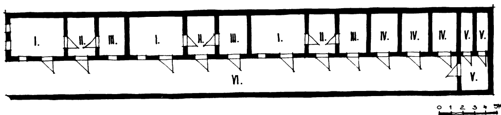
Obr. 13. Podkonice. Slovensko. Dlhý dom s tromi rezidenčnými jednotkami. I – izba, II – pitvor, III – komora, IV – maštaf, V – stodola, VI – dvor. A. Gregorčok Igovän, 1977.
