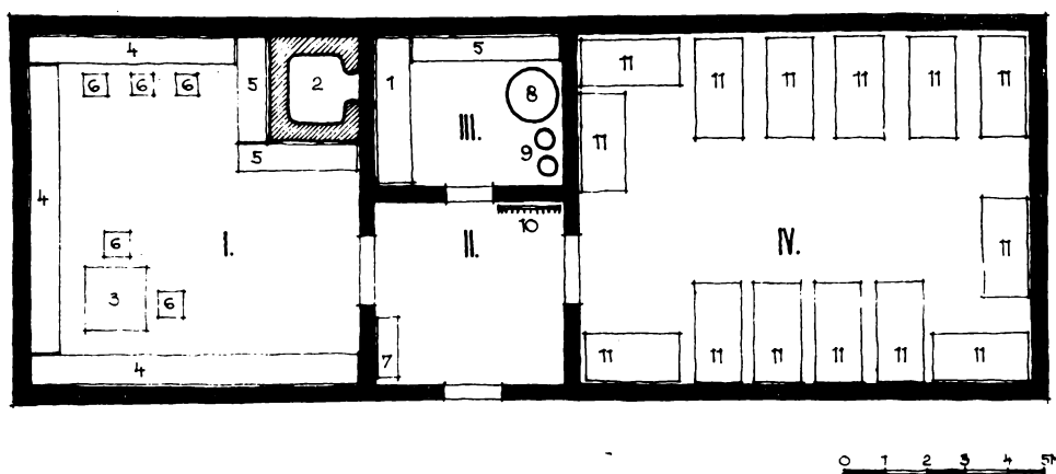
Obr. 1b. Litava, Slovensko. Obytná časť obydlia rodiny Balkovcov: I – chiža (izba), II – pitvor (vstupný priestor), III – čierna kuchyňa, IV – komora na spávanie: 1 – ohnisko, 2 – pec, 3 – stôl, 4 – lavice, 5 – lavičky, 6 – stoličky, 7 – lavička na nádoby s vodou, 8–9 – nádoby na pomyje, 10 – vesiak na odev, 11 – posteľe. J. Botík. 1969.
