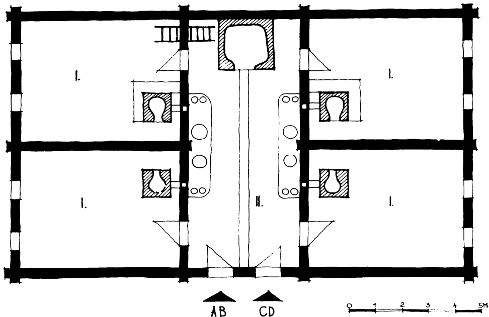
Obr. 12. Štôla. Slovensko. Štvordom so spoločným vstupným priestorom. I – izba, II – pitvor. S. Švecová, 1964.
