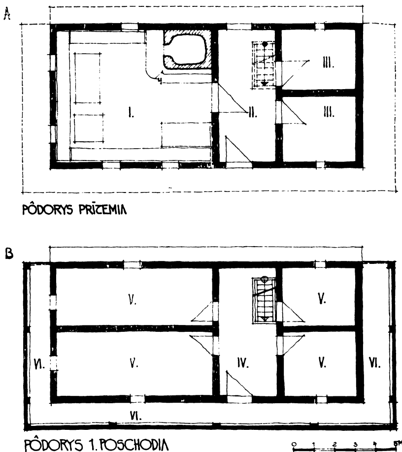
Obr. 3. Čičmany, Slovensko. Obydlie rozšírenej rodiny Petrášovcov: A – Prízemie: I – izba, II – vstupný priestor, III – skladovacie komory; B – Poschodie: IV – predčlenov so schodištom, V – komory na spávanie, VI – pavlač. D. Stránska, 1966.
