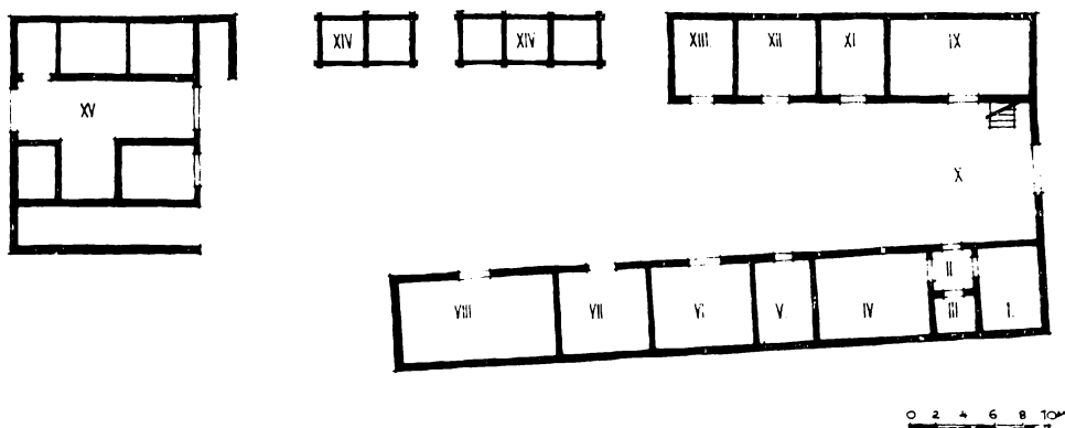
Obr. 1a. Litava, Slovensko. Obydlie rozšírenej rodiny Balkovcov: I – izba, II – vstupný priestor, III – čierna kuchyňa, IV – komora na správanie, V – maštaľ pre kone, VI – maštaľ pre voly, VII – maštaľ pre kravy, VIII – ovčín, IX – komora na skrine s odevom, X – pivnica, XI – komora na potraviny, XII – dielňa, XIII – komora na náradie, XIV – chlievy pre svine a hydinu, XV – stodola so sýpkou na obilie. J. Botík, 1968.
