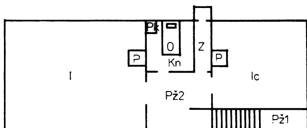
Obr. 8a. Lazini, Chorvátsko. Usadlosť rodiny Domladovac: D – dvor, I – iža (hlavná obytná stavba), K – komore (obytné priestory jednotlivých malých rodín), Kn – chlievy pre hydinu, Pj – stodola, Js – sýpka, Uv – hlavný vchod do dvora, S – senník, Šl – maštal, U – vedľajší vchod do dvora, Sv – chliev pre svine, Kr – maštal pre kravy, G – gánok, Gt – hnojisko, V – maštal pre voly, B – studňa, Vt – záhrada, L – pasienok. D. Švob–F. Petrić, 1929.
