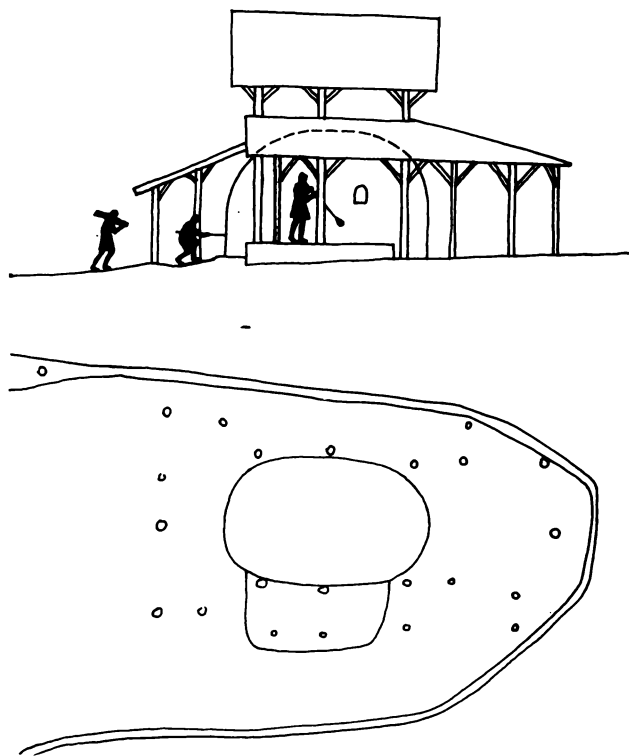
Obr. 2. Řez rekonstruovanou sklářskou hutí z Moldavy I, okr. Teplice a schématický půdorysný plán objektu. (Kresba Ing. arch. P. Chotěbor.)
