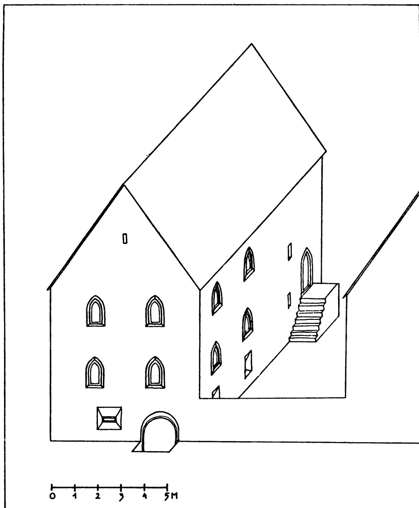
obr. 3. Nálepškova 16 — rekonštrukcia pohľadu na objekt z Nálepčkovej ulice. Objekt je v hmote zachovaný vo výške všetkých podlaží, okenné otvory horných podlaží sú rekonštruované hypoteticky. Rekonštrukcia: M. Zemková.
