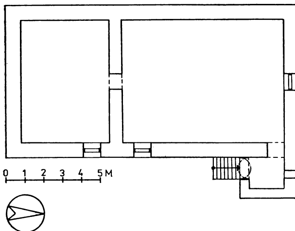
Obr. 10. Prepoštská 11 — rekonštrukcia oboch podlaží objektu z konca 13. storočia. Okno v severnom múre druhého podlažia je rekonštruované hypoteticky. Rekonštrukcia: autorka.
