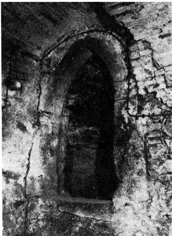
Obr. 5. Kamenný podklenutý pás v spodnom podlaží objektu Nálepková 16, ktorý nesie priečku horného podlažia. Nad vrcholom oblúka je viditeľná pôvodná úroveň podlahy horného podlažia. Klenba je ranorenesančná. Foto: J. Schramek.
