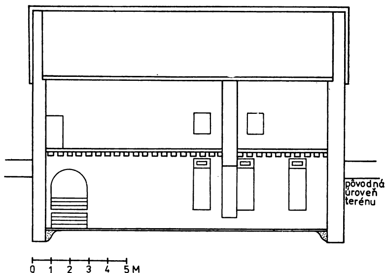
Obr. 11. Prepoštská 11 — rekonstrukce výšky objektu — pozdížný rez. Rekonstrukce: autorka.
