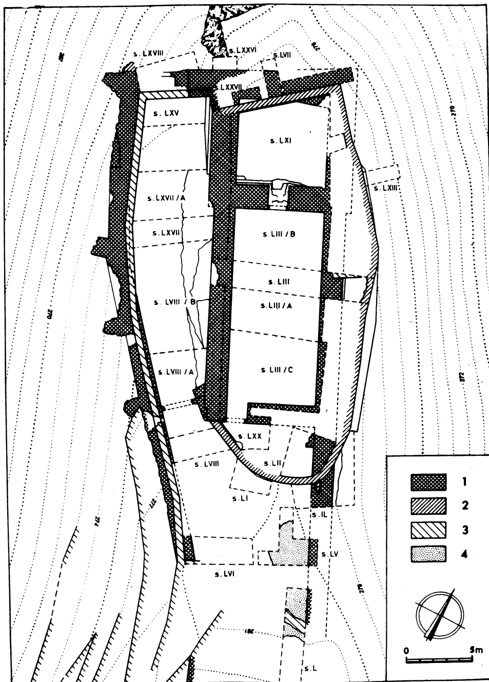
Obr. 2. Křivoklát hrad, okr. Rakovník. Bollwerk a jeho nejbližší okolí s odkrytými pozůstatky manského domu. 1 — zdivo manského domu a přilehlých fortifikací (okolo 1400 ), 2 — zdivo vladislavské přestavby, 3 — subrecentní a recentní zdíva, 4 — maltová podlaha stavby v prostoru krčku před manským domem. Kresba J. Tájek.
