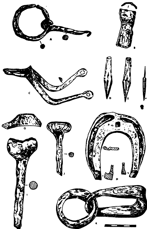
Obr. 10. A — uditko, B — část brnění rukavice, C — ostraha, D—F — hroty šípů, G — ozub podkovy, H — podkova, I—J — zákolníky, K — závěs vah. Materiál z různých uhledlostí.
