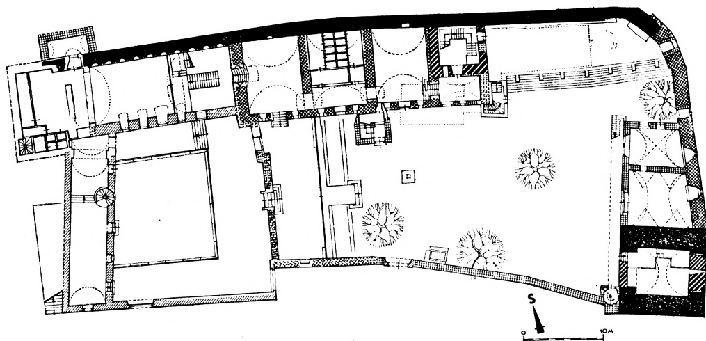
Obr. 8. Půdorys přízemí areálu po úpravě na Dům čsl. dětí v letech 1960–63 ve stavebně historické analýze – legenda viz obr. 7 (F. Kašíčka)
