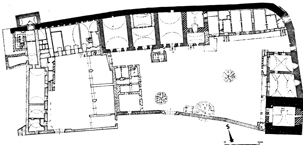
Obr. 7. Půdorys přízemí areálu před r. 1960 – rekonstrukce stavebně historické analýzy. Černě označeno románské zdivo Černé věže a hradby, černými pruhy mladší románská zazdívka brány a zdivo věže v purkrabství, šikmé mřížky – zdivo gotické, mřížky kolmé ke konstrukci – renesanční, šikmá šrafa – zdivo barokní, ostatní – klasicistní a novodobé. Přerušované pojednání značí zařazení hypotetické (F. Kašíčka).
