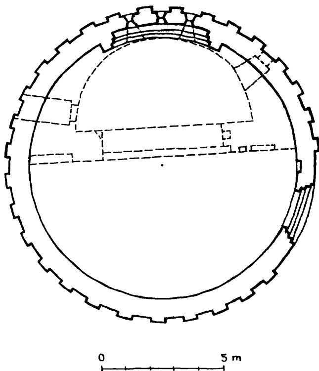
Obr. 5. Ideální rekonstrukce původní koncepce půdorysu rotundy v Šivetících (M. Rađová).
