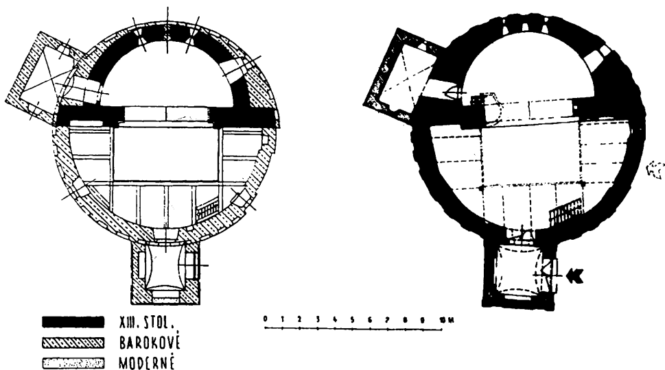
Obr. 2. Půdorys rotundy v Šivetíciach podle V. Mencla a půdorys z archivu katedry teorie a dějin architektury SVŠT v Bratislave z r. 1977.
